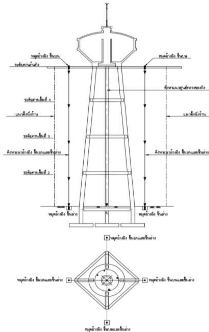
รูปที่ 65 การกำหนดมุมอ้างอิง ที่ระดับพื้นชั้นล่าง และชั้นบน
