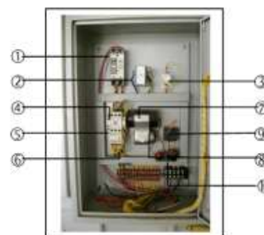
ลักษณะภายในตู้ควบคุม เครื่องสูบน้ำแบบซับเมอร์ส
