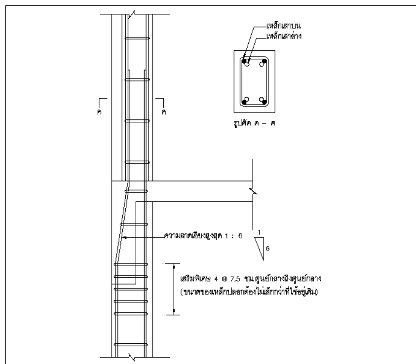
รูปที่ 31 การต่อเหล็กเสากรณีเสามีหน้าตัดไม่เท่ากันศูนย์เอียงกัน
