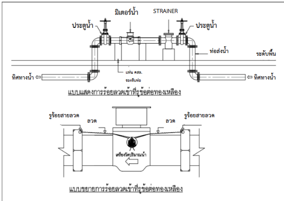
1) แบบขยายการร้อยลวดทองแดงที่รูข้อต่อของเหล็องของเครื่องมือวัดปริมาณน้ำ
