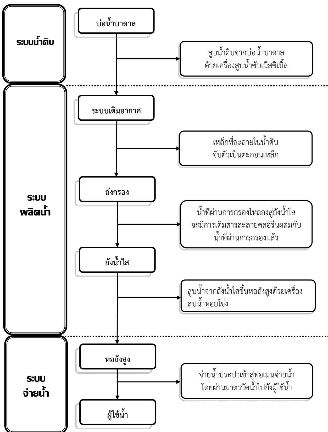
รูปที่ 1 กระบวนการผลิตน้ำประปา
