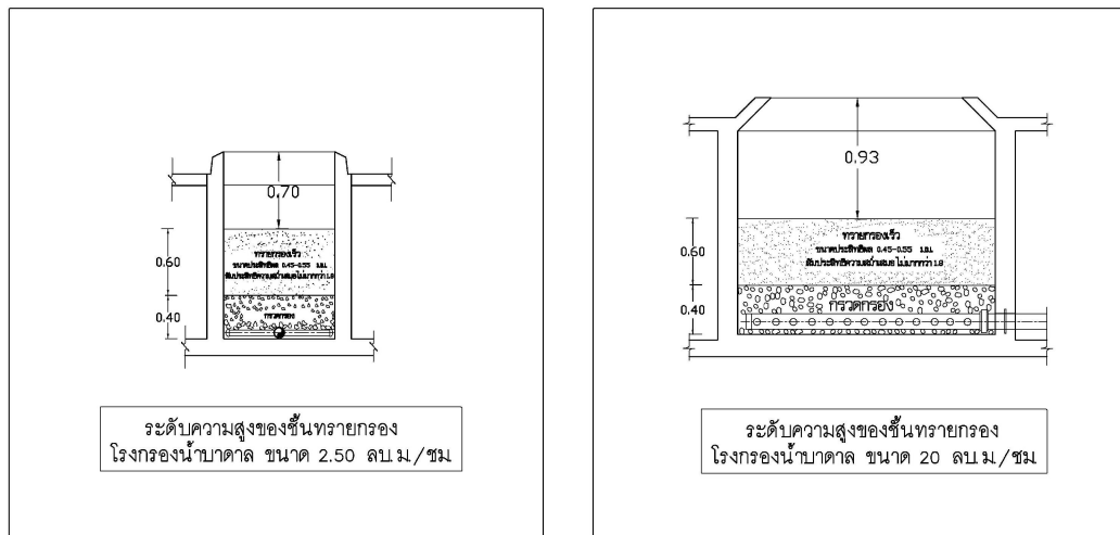
รูปที่ 23 ทรายนกรองและระดับความสูงของทรายนกรองที่ถูกต้อง
